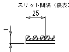
長尺型断面図
