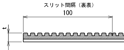
角型断面図
