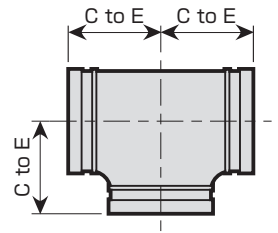
No. 002 ショートチーズ
